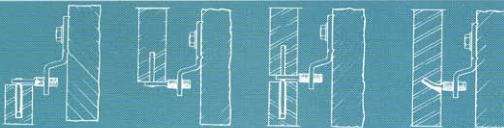
Attache ponctuelle chevillée de retenue
